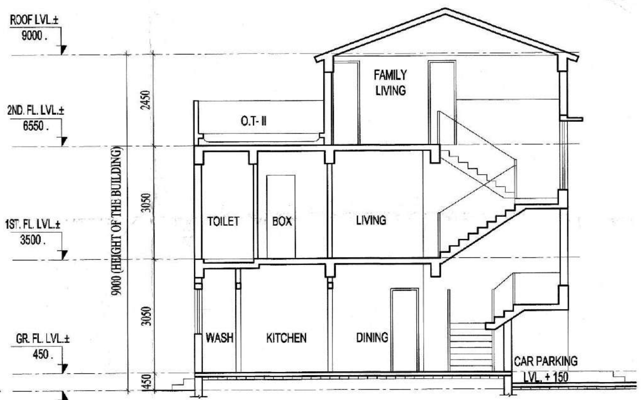
SECTION D-D
